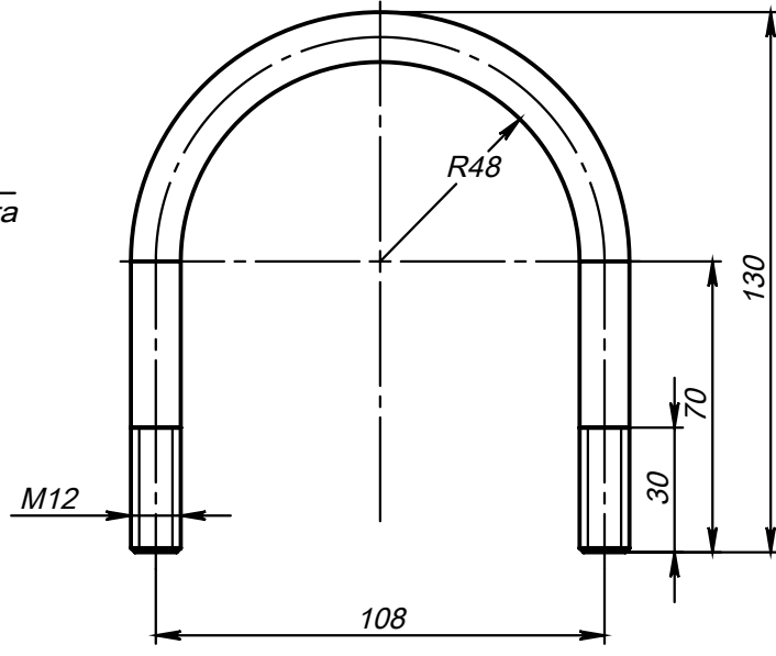
Поз.5 (Хомут)
