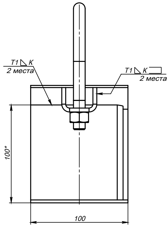
Поз.3 (Пожемент)
